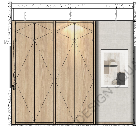
B-109 : WARDROBE ELEVATION 07
