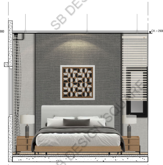
B-211 : WALL BEDHEAD ELEVATION 19
